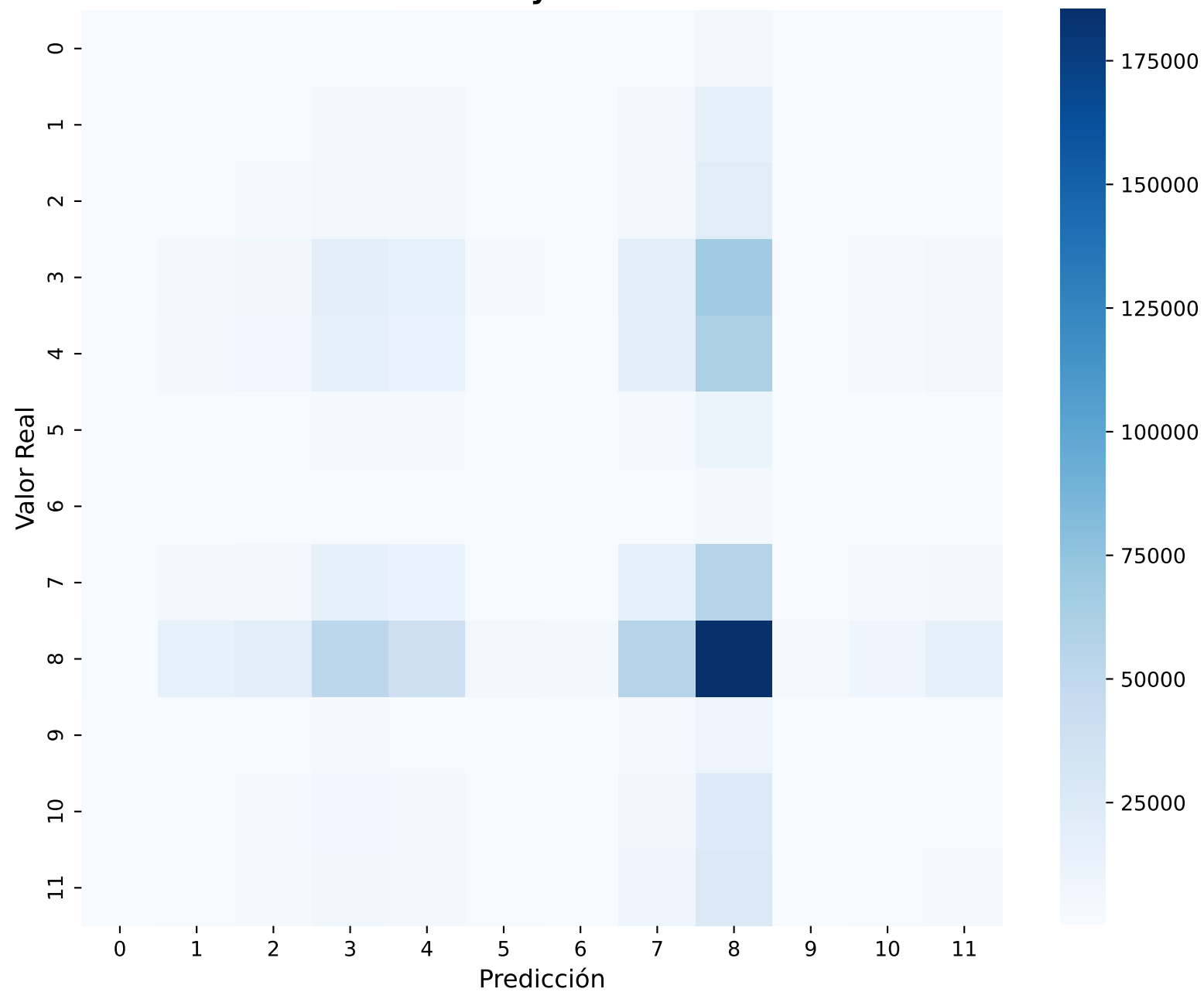
Matriz de Confusión - MobileNetV2 (Best Model)
